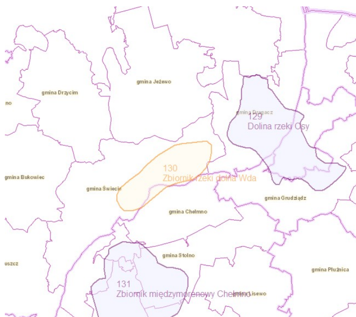
Rysunek 7 Główne zbiorniki wód podziemnych
